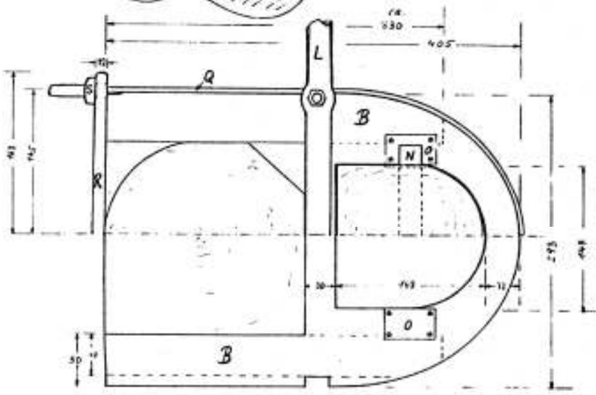
Kälber und Stengefuß-Bettung Maßstab 1:2
